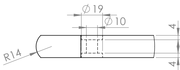
DÉTAIL A ECHELLE 1 : 2
