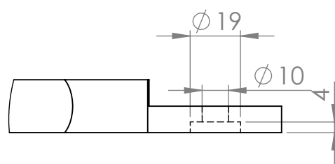
DÉTAIL B ECHELLE 1 : 2
